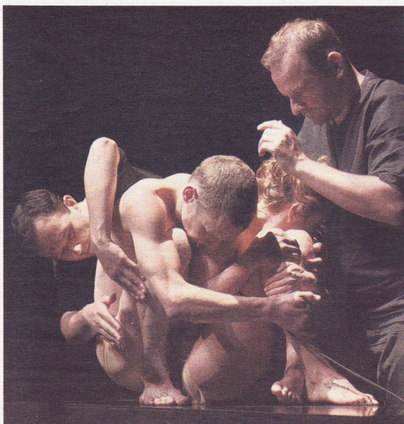
Huid.
